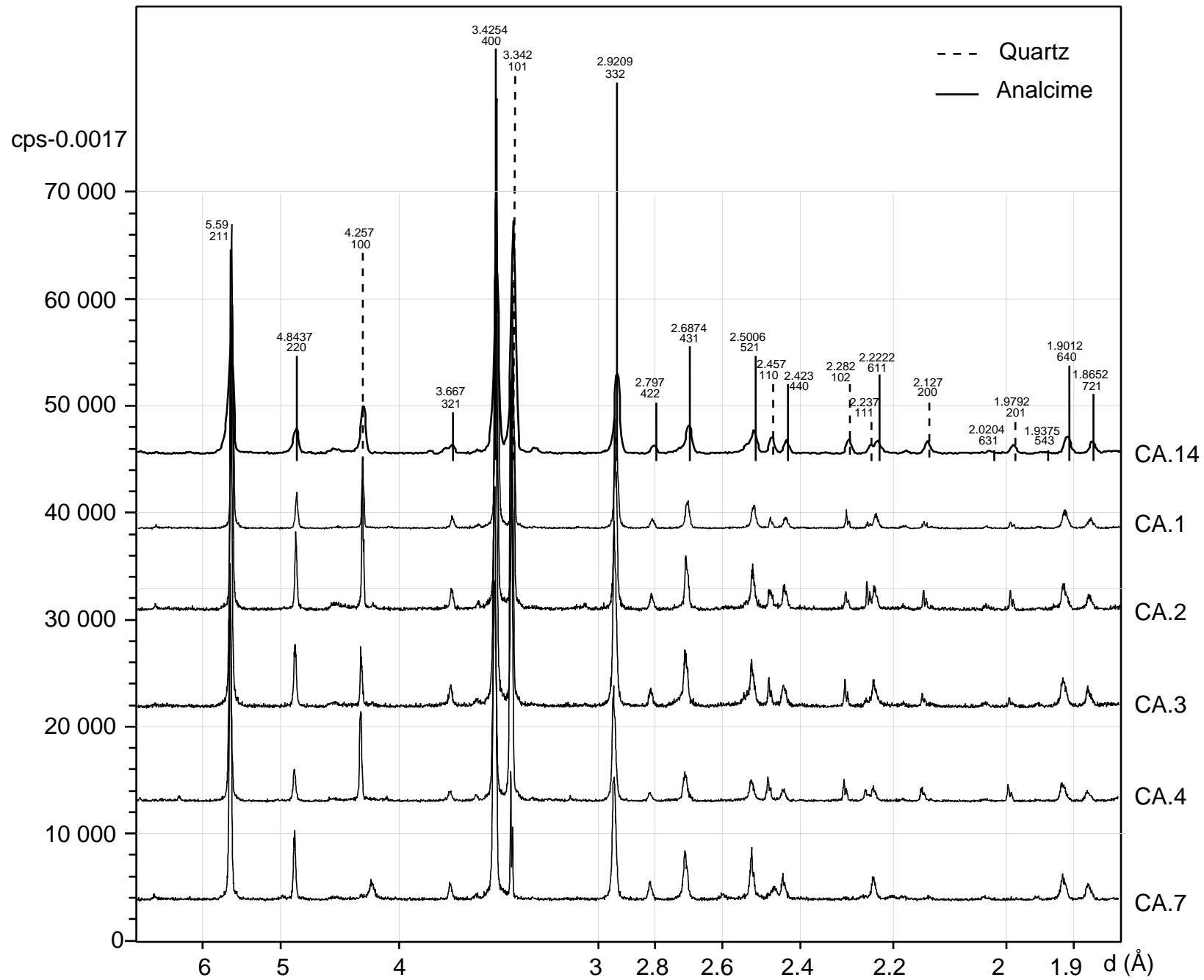
Figure S-3.a : Diffractogrammes DRX des échantillons contenant essentiellement de l'analcime et du quartz.
