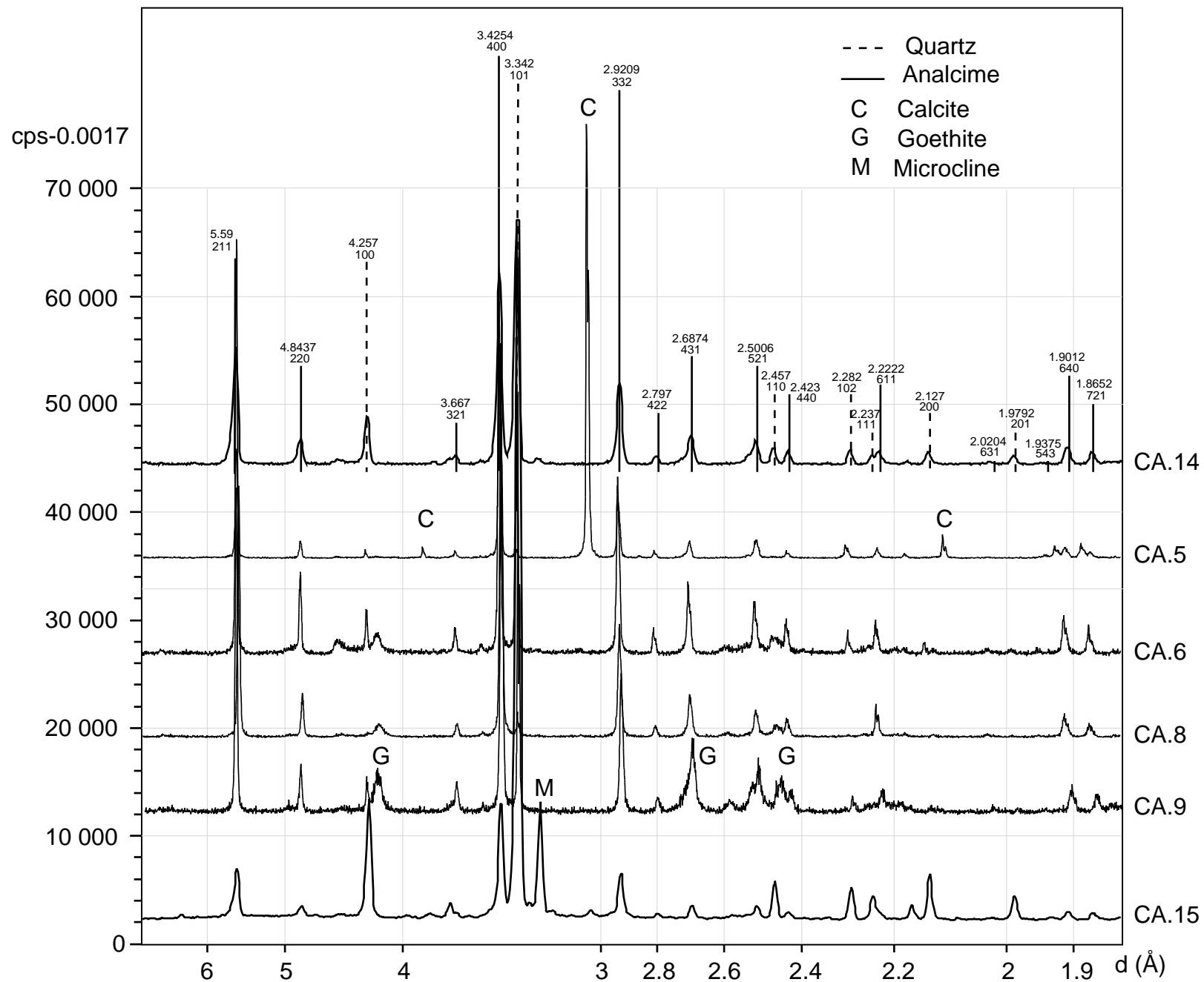
Figure S-3.c : Diffractogrammes DRX des échantillons contenant d'autres phases cristallines en dehors de l'analcime et du quartz.
