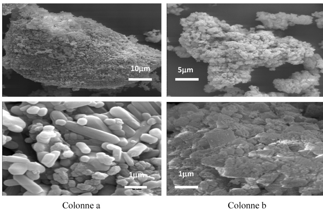
Fig. 4. Clichés de MEB, à différents agrandissements, de PN tout seul (colonne a) et V/PN (1 mmol) calciné à 800 °C (colonne b).
