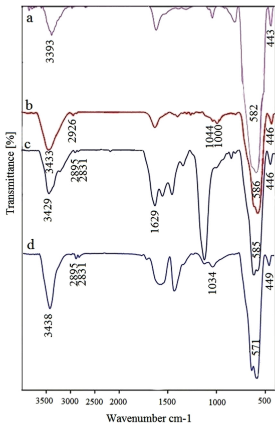
Fig. 4. FT-IR spectra of \text{Fe}_3\text{O}_4 (a), Cl-MNPs (b), SMU-MNPs (c) and Pd-SMU-MNPs (d).
