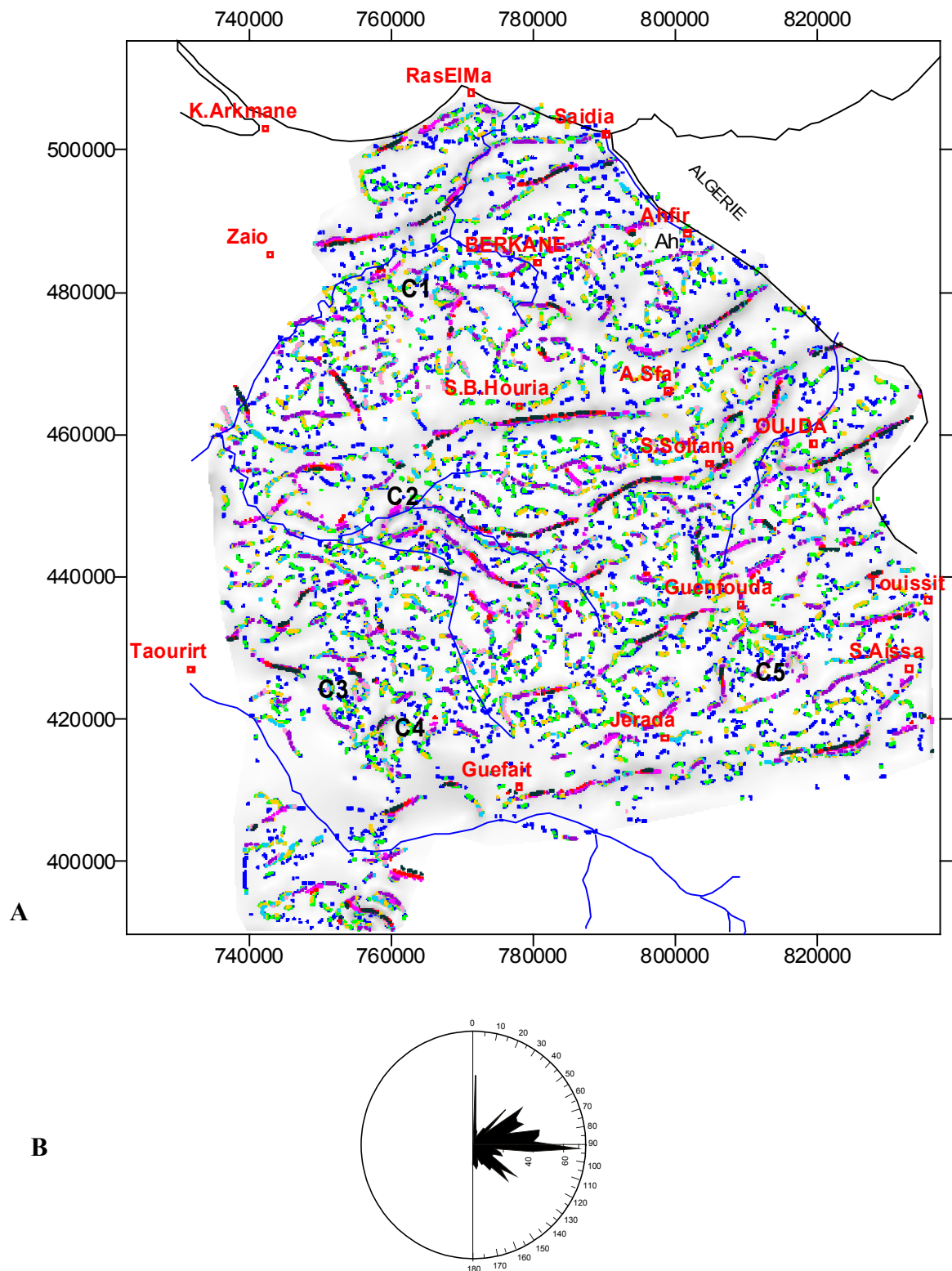
Fig.3 Superposition des maxima du gradient horizontal obtenus sur la carte de Bouguer et sur les cartes prolongées vers le haut à différentes altitudes (A) et rosace des fréquences des alignements interprétés comme étant des failles (B). ● maxima sur la Bouguer ; ● 250m ; ● 500m ; ● 750m ; ● 1000m ; ● 1500m ; ● 2000m ; ● 2500m ; ● 3000m.
