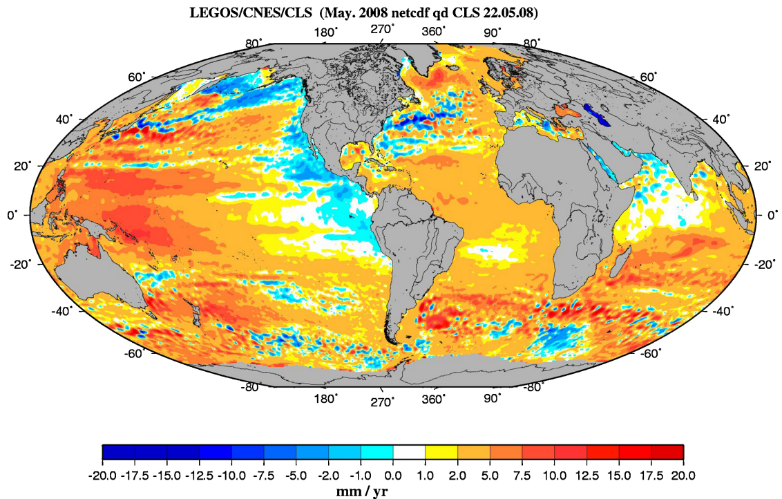
Fig. 3. Geographical distribution of linear sea level trends computed over 1993–2008 from multisatellite altimetry. Distribution géographique des vitesses de variation du niveau de la mer entre 1993 et 2008 basées sur les données altimétriques multisatellites.
