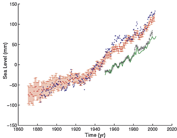
Fig. 2. Sea level curve for the 20th century based on different tide gauges data and reconstruction analyses. Red dots: data from [11]; Blue dots: data from [19]; Black dots: data from [16]; Green curve. 3 Évolution du niveau de la mer mesurée au cours du xx e siècle d'après diverses reconstructions utilisant les enregistrements marégraphiques. Points rouges : données de [11] ; points bleus : données de [19] ; points noirs : données de [16] ; courbe verte. 3
