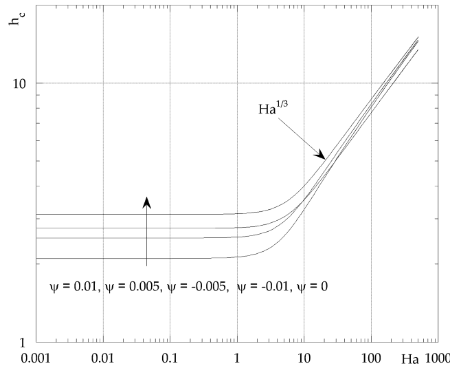
Fig. 3. Variation de h_c avec Ha pour Pr = 0.01 , Le = 0.01 et différentes valeurs de \psi . Fig. 3. Variation of h_c with Ha for Pr = 0.01 , Le = 0.01 and different values of \psi .
